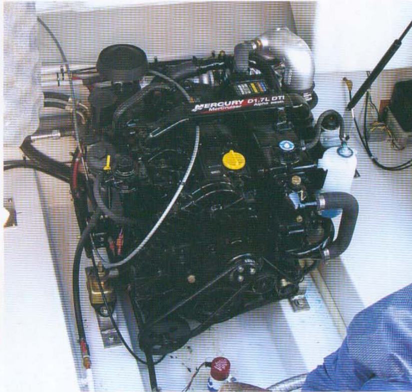
116 hk Mercruiser 1,7 liter er let at komme til fra alle sider.
