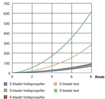
Modstand (N)
